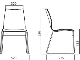
S290L SL SLED
