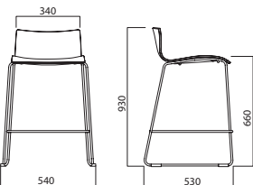
SG290L SL SLED STOOL
