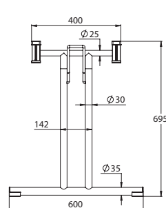
Piedino fisso Fixed foot
