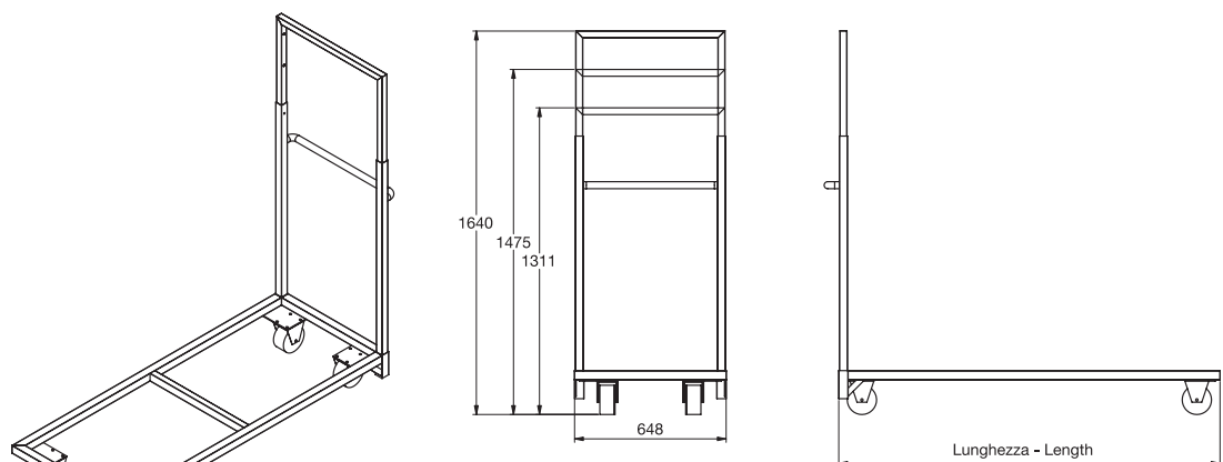
CRTAV-140 CARRELLO PER TAVOLI - TABLE TROLLEY L=140 ZINC CRTAV-160 CARRELLO PER TAVOLI - TABLE TROLLEY L=160 ZINC
