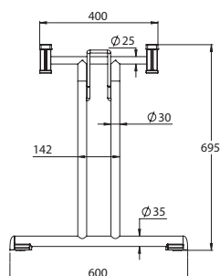
Piedino regolabile Adjustable foot
