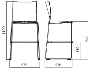
SG220L SLED STOOL
