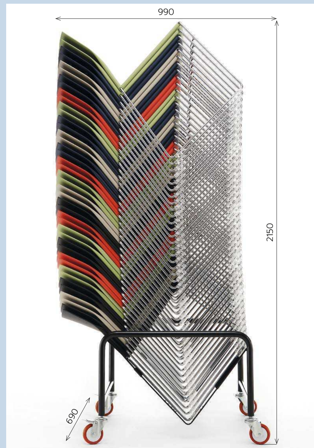
Impilabilità, su carrello con inclinazione a 45° fino a 45 sedie High density stacking 45 chairs on a trolley, tilting up to 45°
